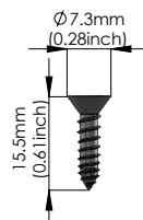
SCREWS (SUS 304)
